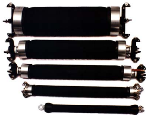
Packer ad alta pressione per il posizionamento della guaina inossidabile RIVA
